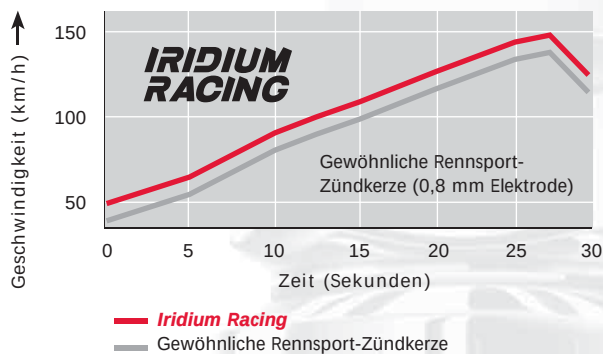
Verbesserte Beschleunigung Data: In-Company Comparison
