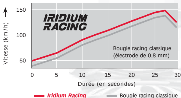
Accélération améliorée Data: In-Company Comparison
